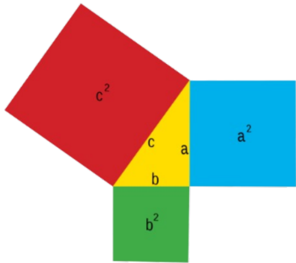
피타고라스의 정리
