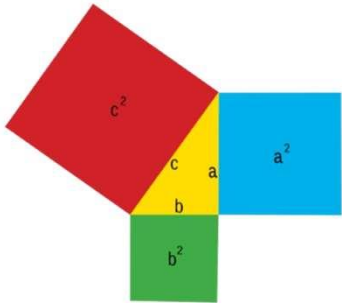
피타고라스의 정리
