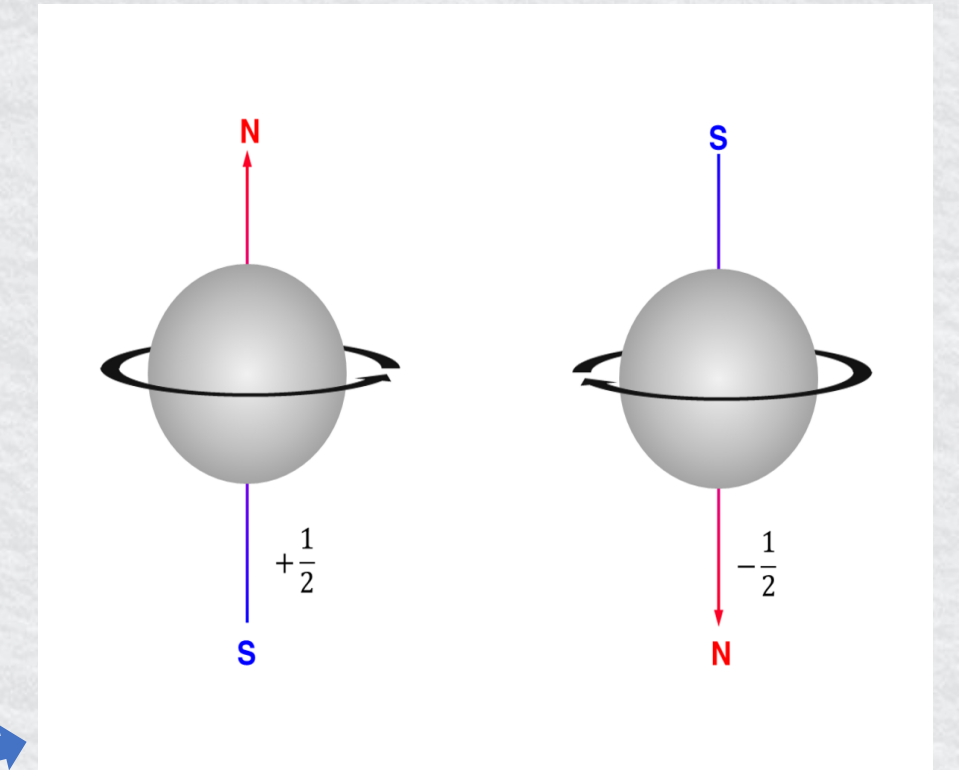
전자의 회전량 +1/2 와 -1/2
