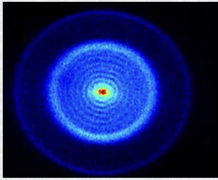
수소원자 2017년 촬영
