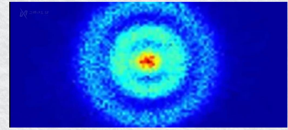
수소원자 2014년 촬영
